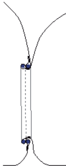
Coupe sur connexion de deux gonflables en simple membrane
